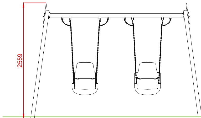
ALZADO
