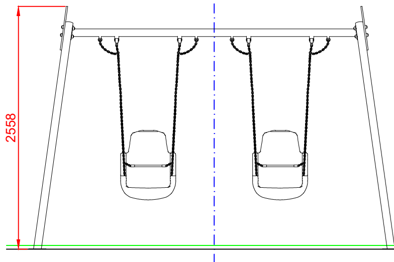
ALZADO
