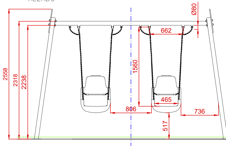
ALZADO
