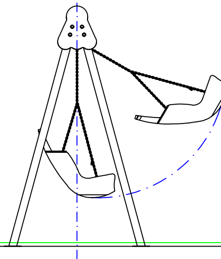
PERFIL
