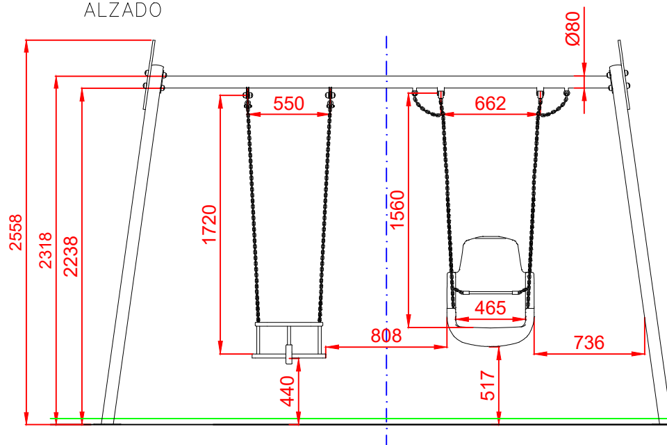
ALZADO
