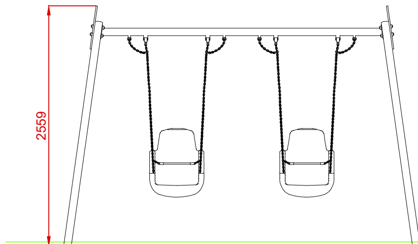
ALZADO
