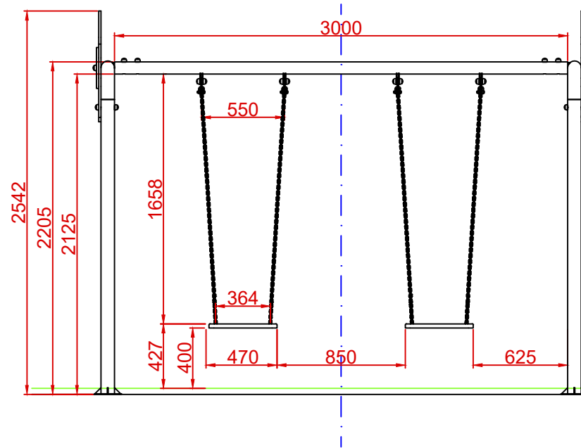
ALZADO
