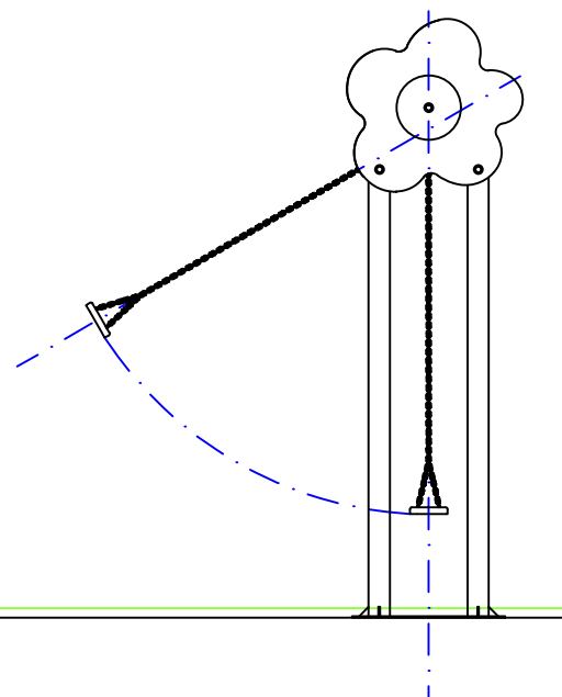
PERFIL
