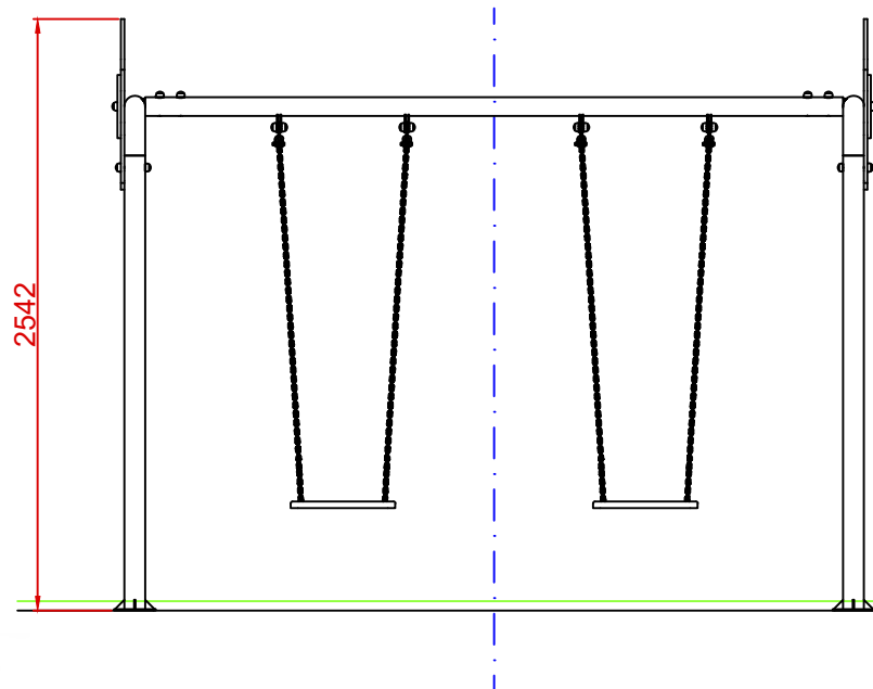
ALZADO
