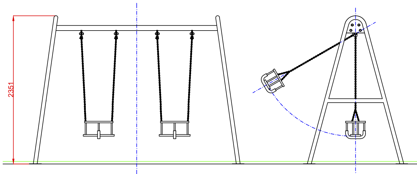
ALZADO
