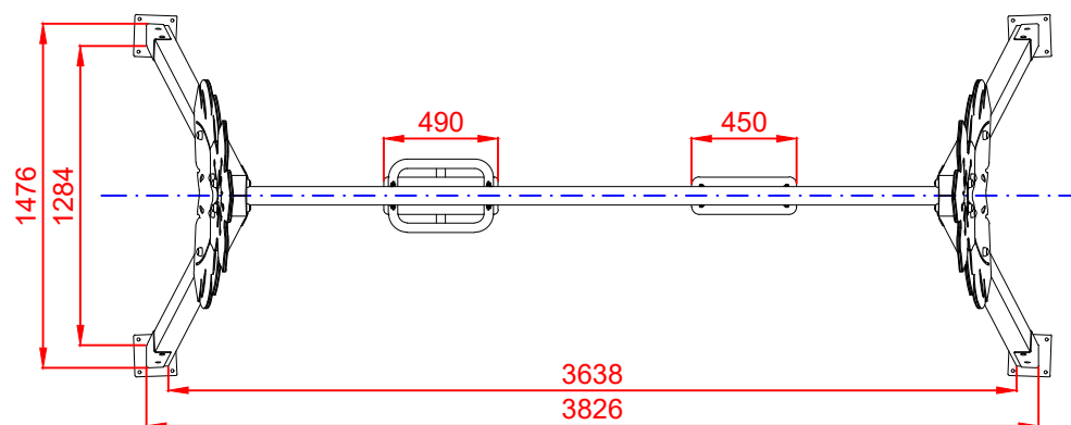
PLANTA
