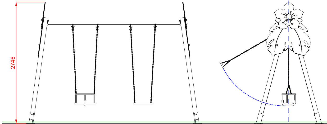
ALZADO
