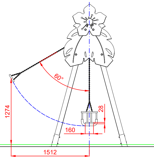
PERFIL IZQUIERDO
