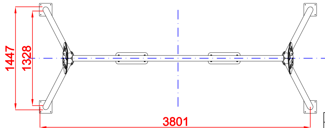
PLANTA
