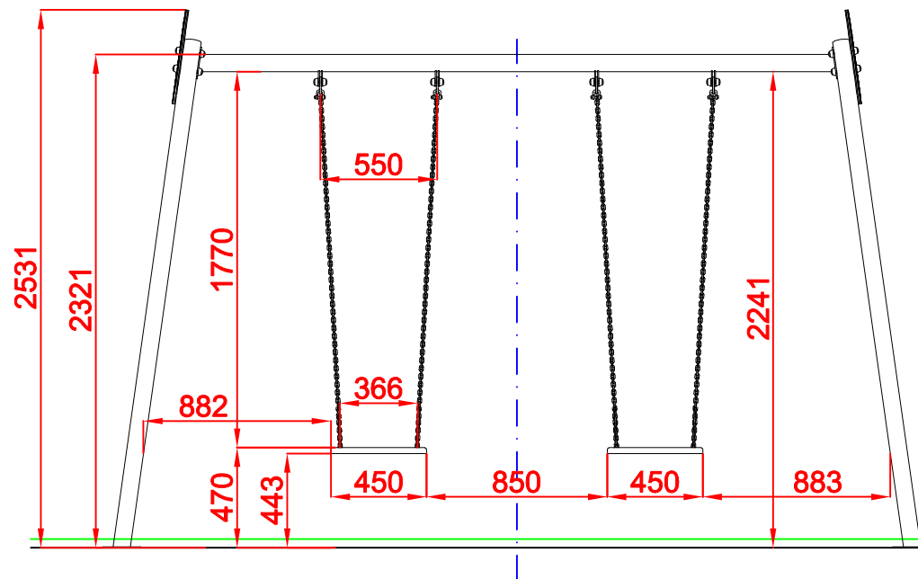
ALZADO
