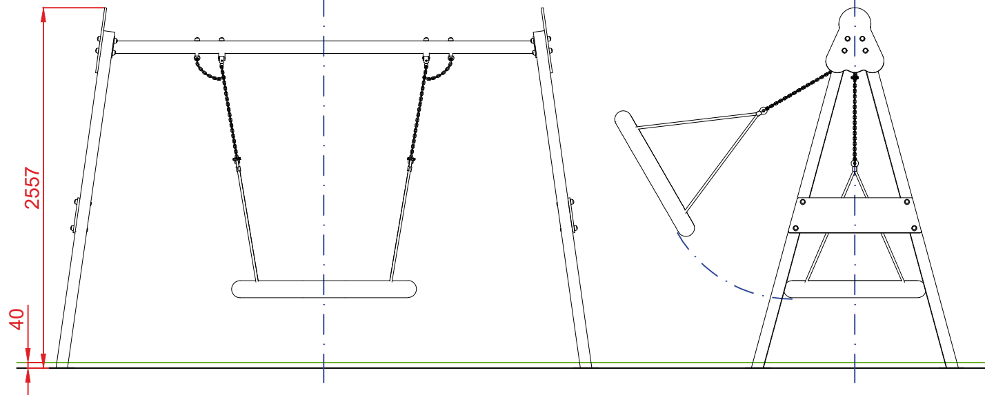
ALZADO
