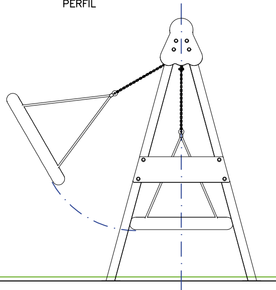
PERFIL
