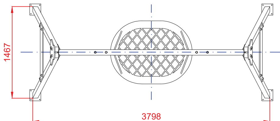
PLANTA
