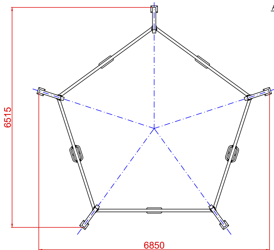
PLANTA
