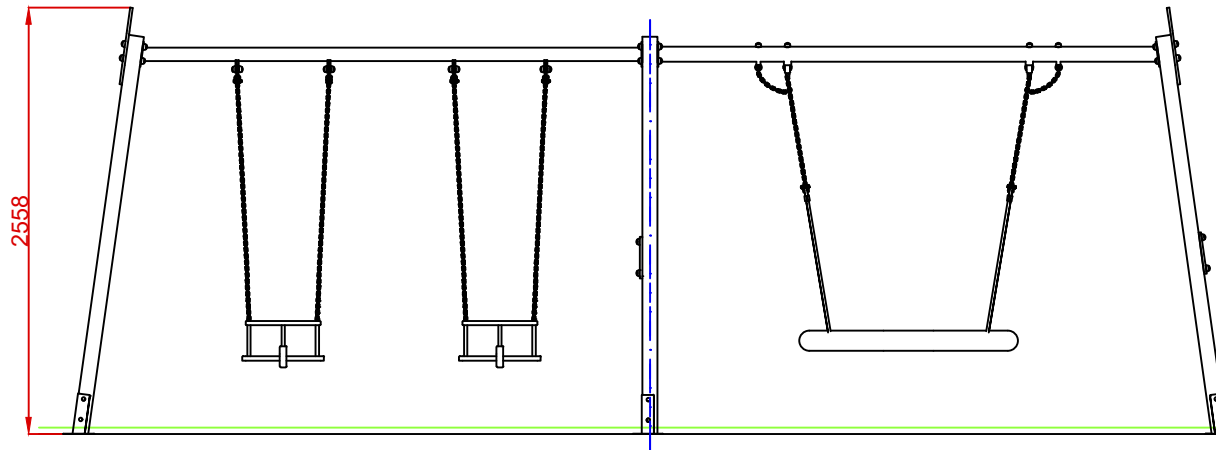
ALZADO
