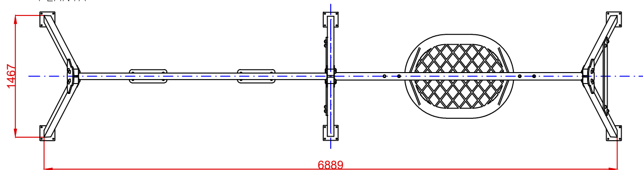
PLANTA
