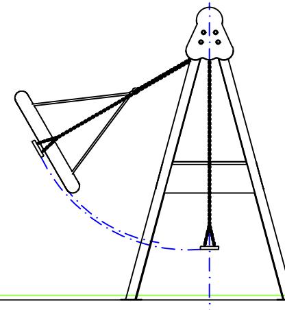
PERFIL
