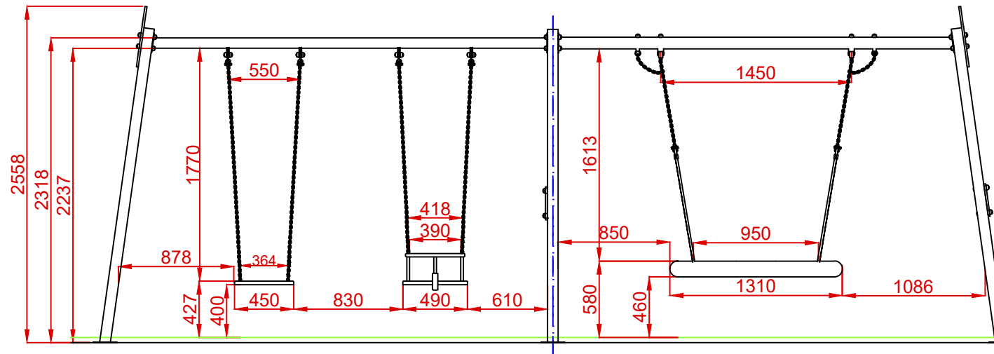
ALZADO
