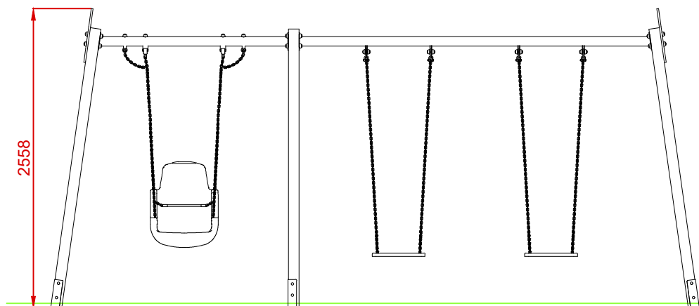
ALZADO
