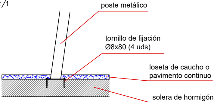
ESQUEMA DE CIMENTACIÓN EN HORMIGÓN E: 2/1
