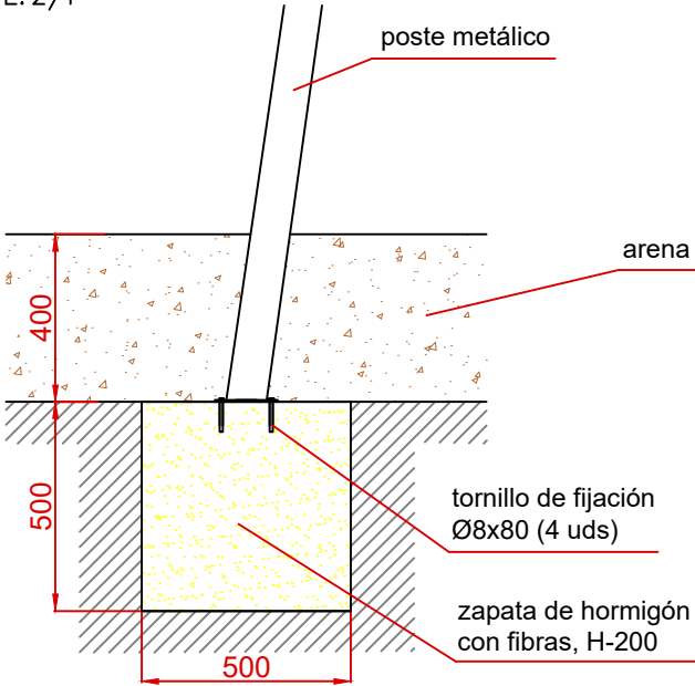
ESQUEMA DE CIMENTACIÓN EN ARENA E: 2/1
