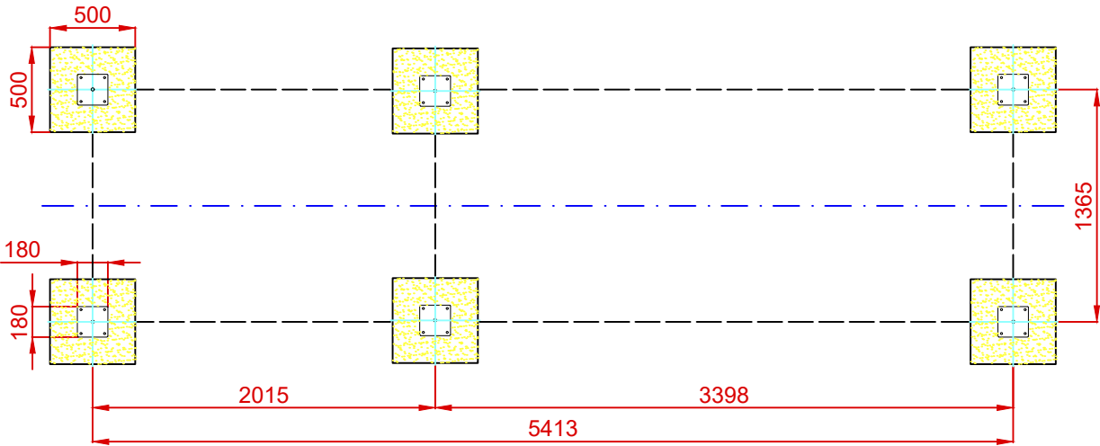
PLANTA CIMENTACIÓN
