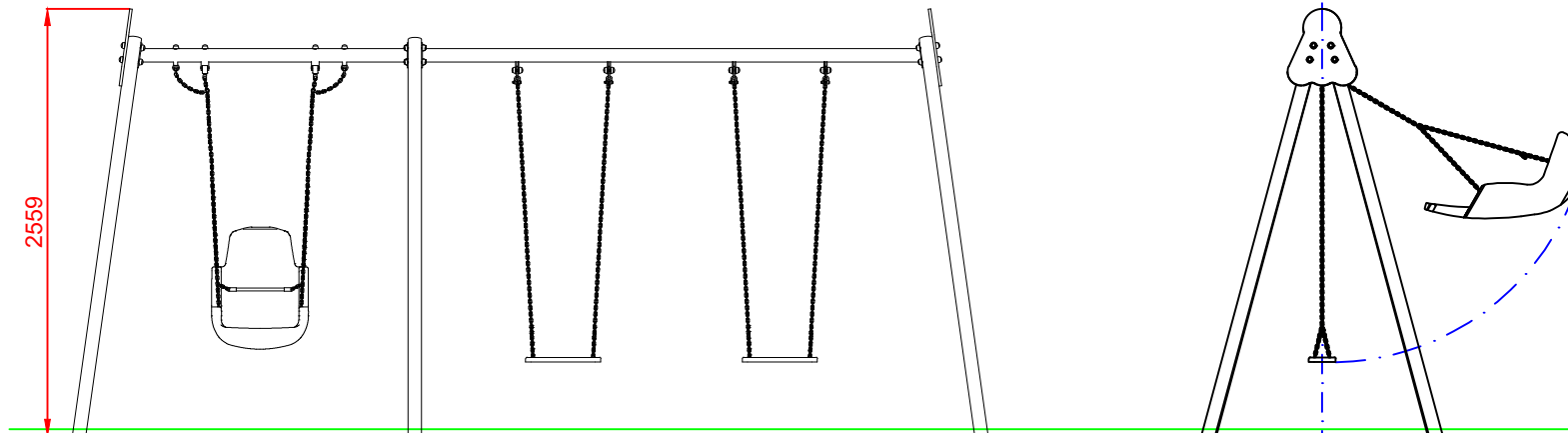
ALZADO
