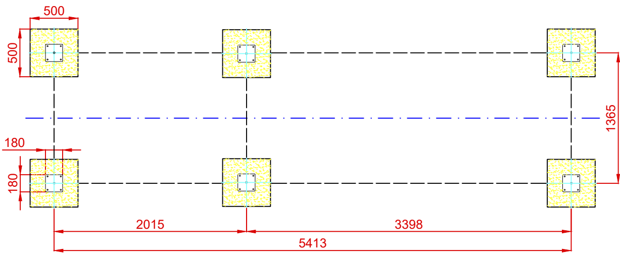
PLANTA CIMENTACIÓN
