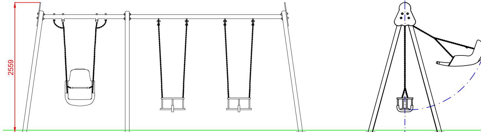
ALZADO
