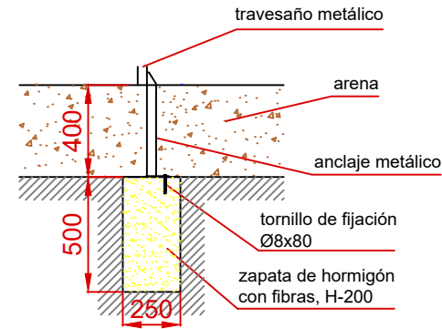
ESQUEMA DE CIMENTACIÓN EN HORMIGÓN
