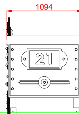
PERFIL IZQUIERDO
