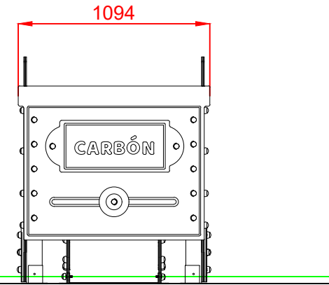
PERFIL IZQUIERDO
