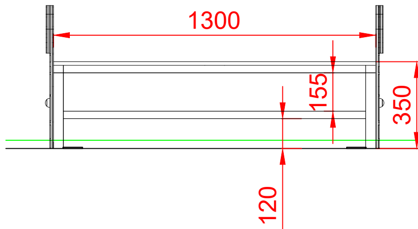
ALZADO
