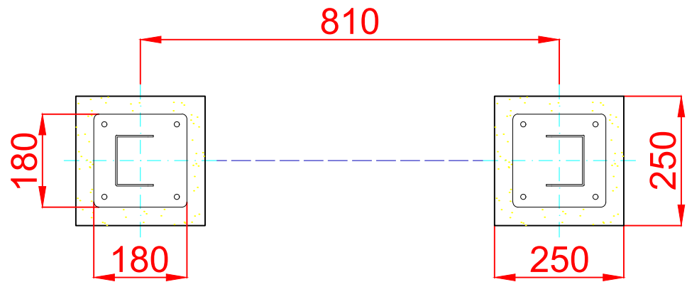
PLANTA CIMENTACIÓN E: 2/1
