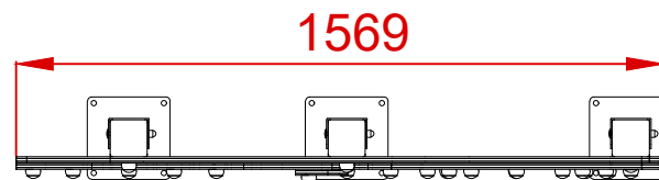
PLANTA
