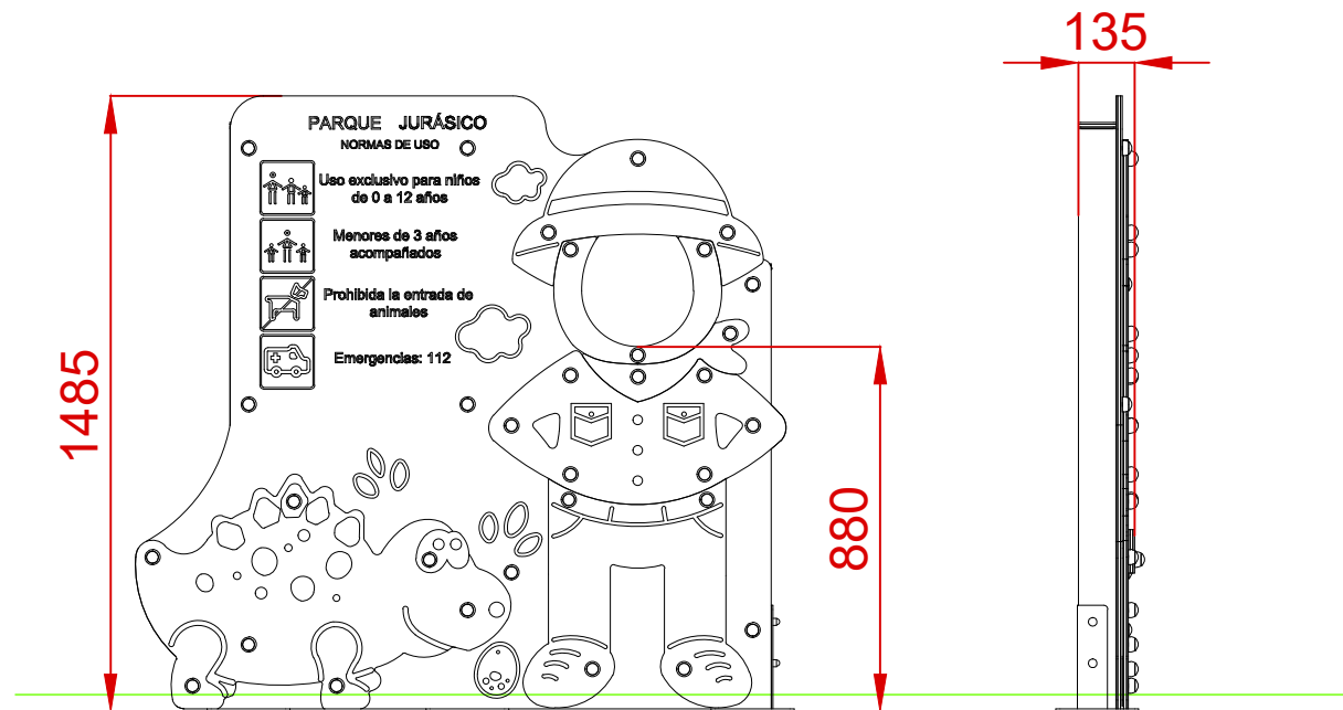
ALZADO
